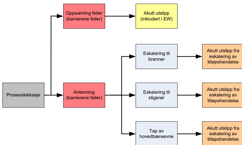
Figur 13 Scenariobeskrivelse prosesslekkasjer 5
