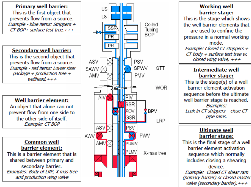
Figur 18 Beskrivelse av de ulike barriereelementene i en brønn (Ref. 44)
