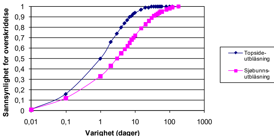
Figur 16 Varighetsfordeling
