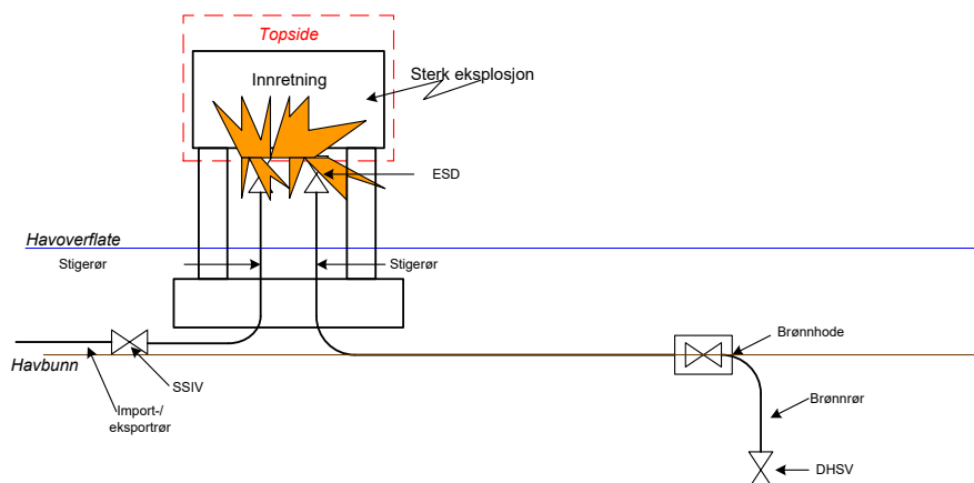
Figur 10 Sterk eksplosjon topside, som ødelegger stigerørs ESD-ventil
