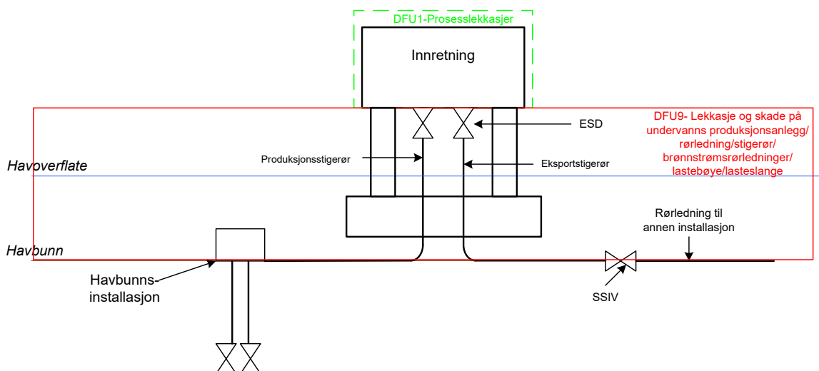
Figur 12 Skille mellom prosesslekkasjer (DFU1) og hendelser knyttet til undervannsproduksjonsanlegg/rørledninger/stigerør/brønnstrømsrørledninger/lastebøyer/lasteslange (DFU9-10)
