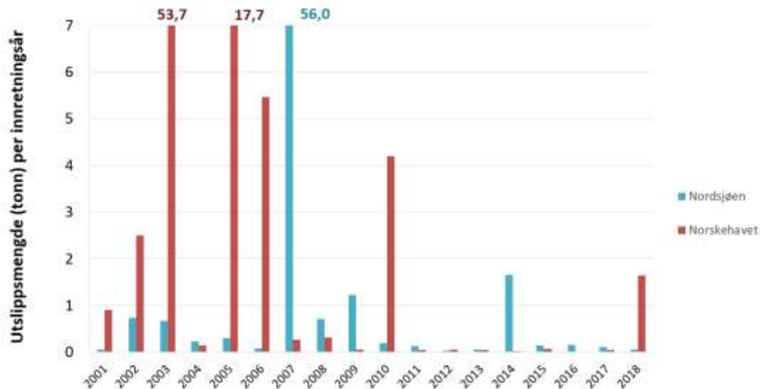
Figur 17 Utslippsmengde for råolje, havområder
