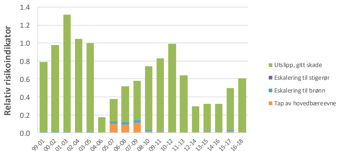
Figur 50 Potensiell utslippsmengde basert på skader og lekkasjer knyttet til stigerør, rørledning og undervannsproduksjonsanlegg 6 norsk sokkel
