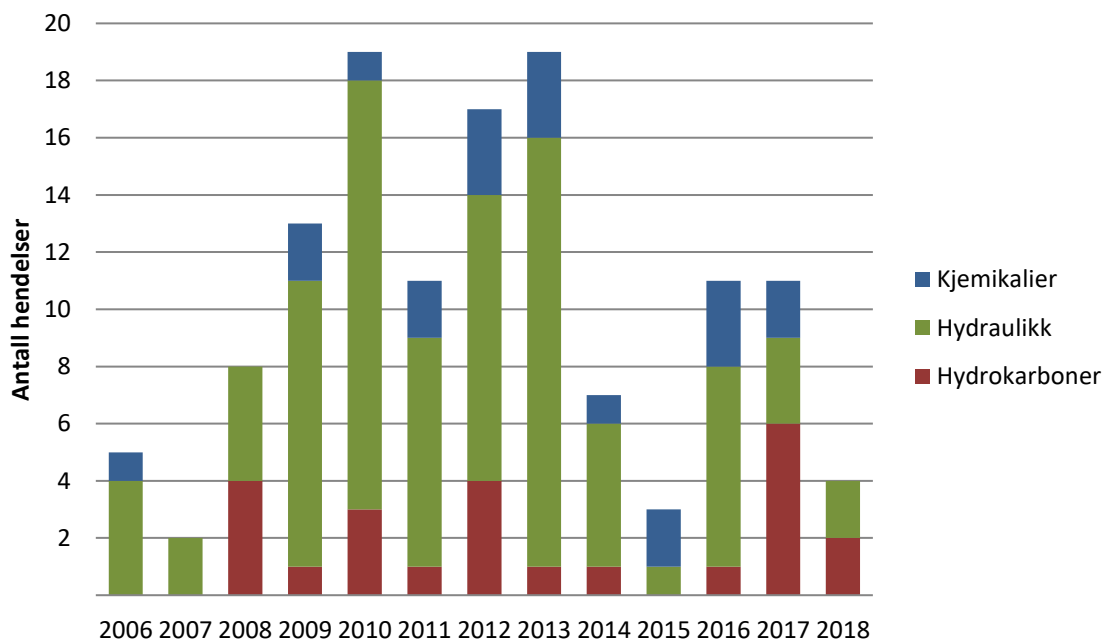
Figur 67 Antall inntrufne akutte utslipp fra havbunnsinnretninger per år, 2006-2018
