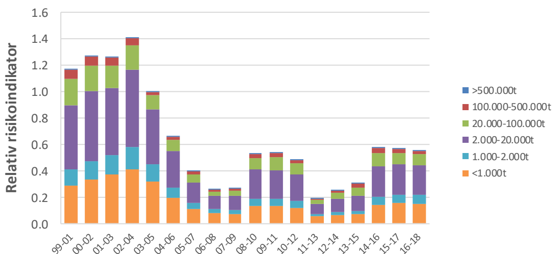
Figur 37 Potensielt antall akutte råoljeutslipp basert på brønnkontrollhendelser, norsk sokkel
