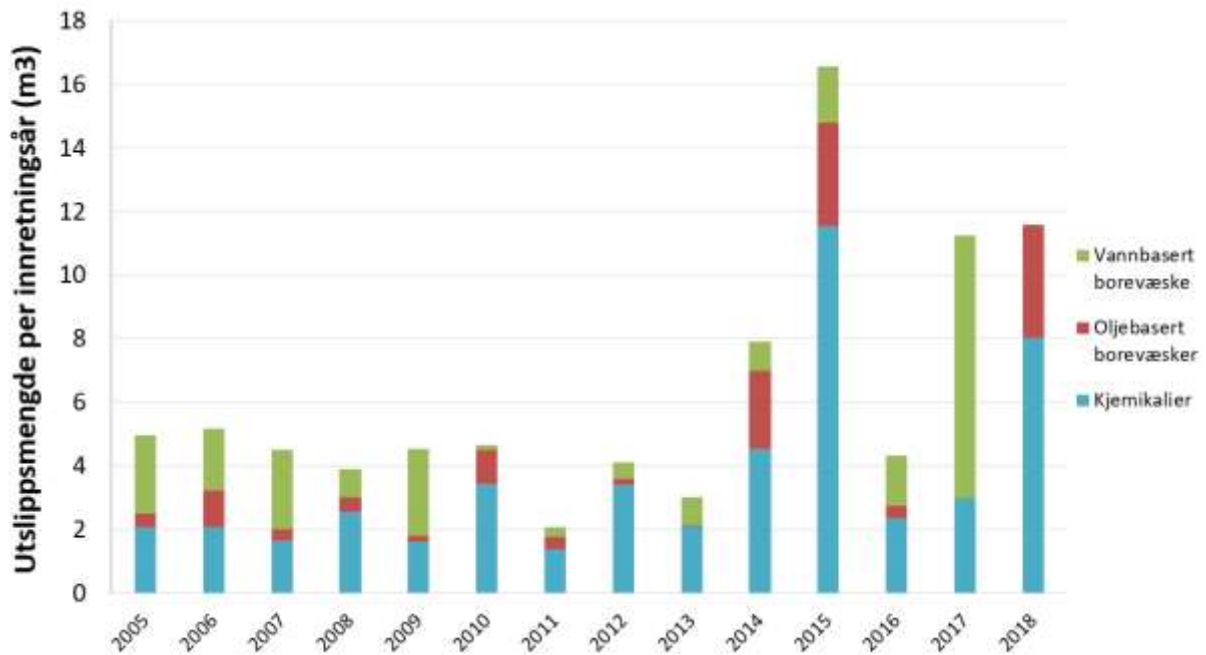
Figur 28 Utslippsmengde per kjemikalietype, norsk sokkel 2005-2018
