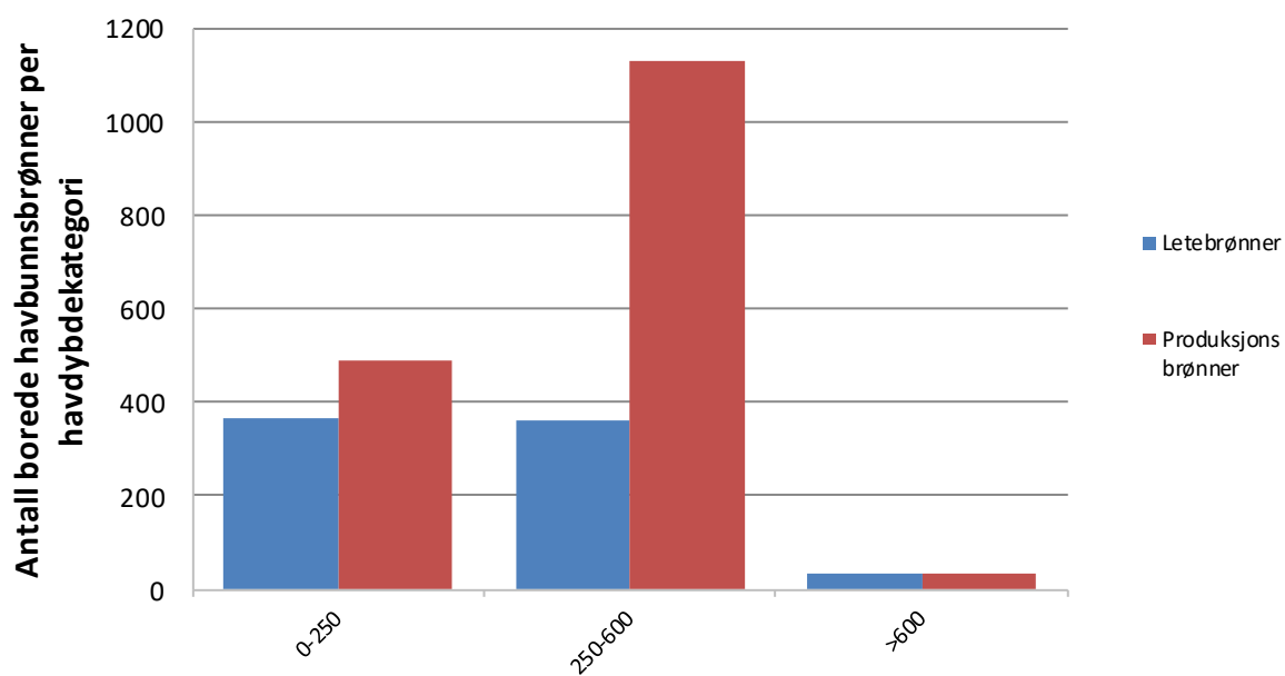
Figur 7 Antall borede havbunnsbrønner, 1999-2018.
