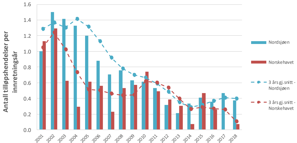
Figur 56 Antall tilløpshendelser, havområder
