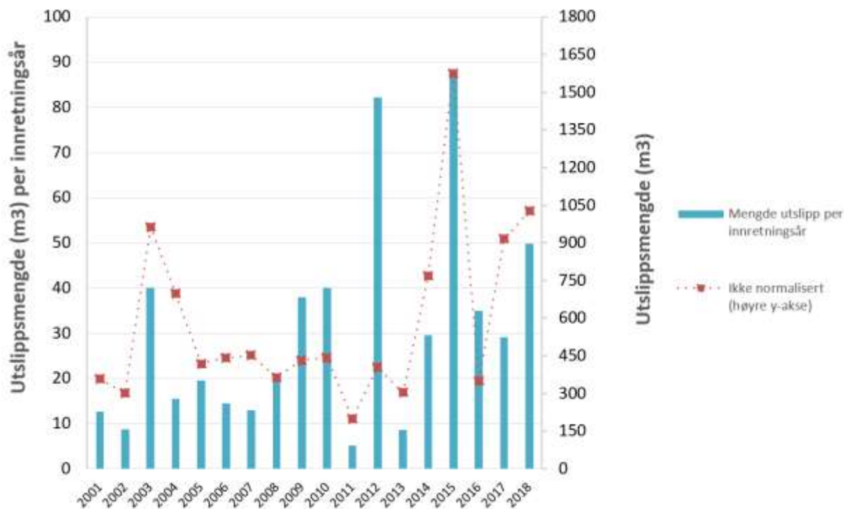
Figur 25 Utslippsmengde for kjemikalier, norsk sokkel
