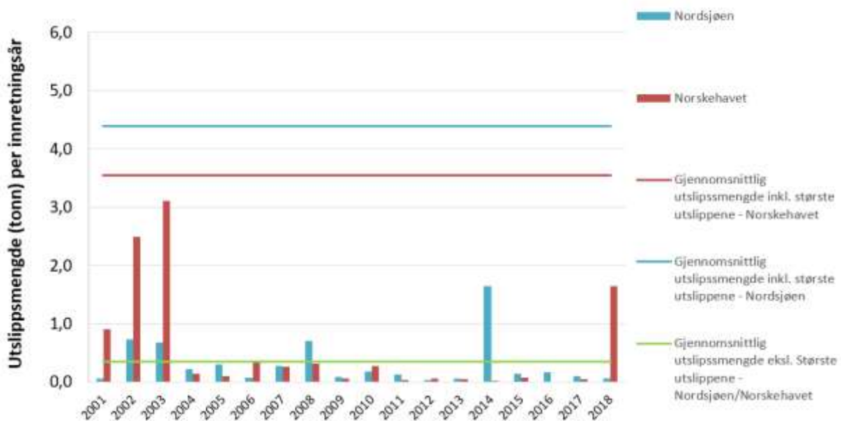
Figur 18 Hendelser med utslippsmengde under 50 tonn, (råolje)
