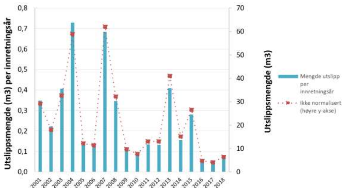
Figur 21 Utslippsmengde for andre oljer, norsk sokkel
