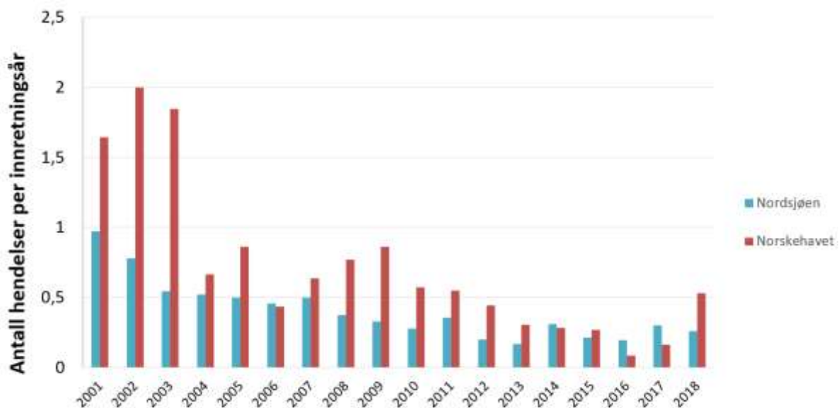
Figur 15 Antall hendelser, råolje, havområder
