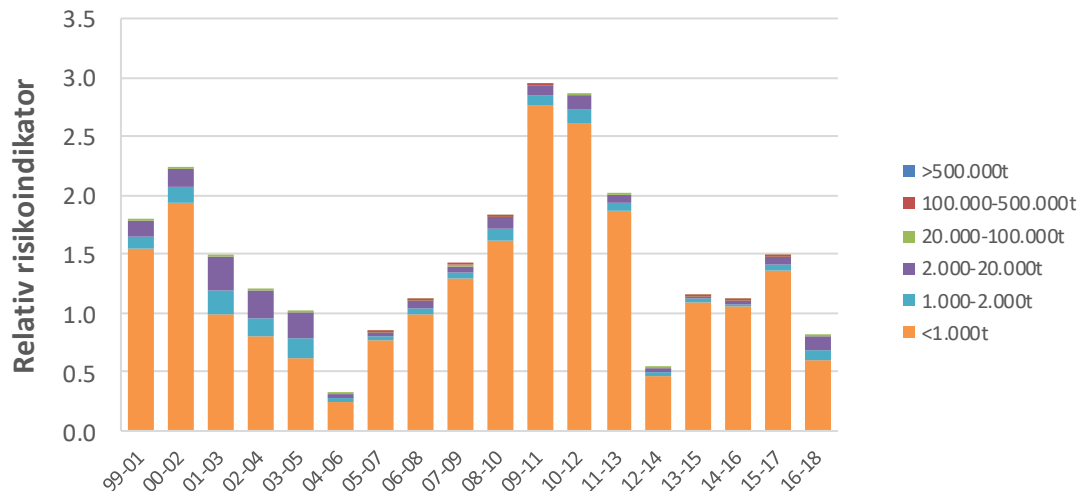
Figur 49 Potensielt antall akutte råoljeutslipp basert på skader og lekkasjer knyttet til stigerør, rørledning og undervannsproduksjonsanlegg 6 , norsk sokkel
