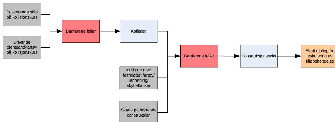
Figur 17 Scenariobeskrivelse konstruksjonsskader 10
