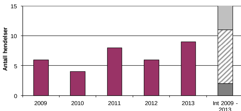
Figur 3 Illustrasjon av observerte verdier for en hendelse og prediksjonsintervall ("int")
