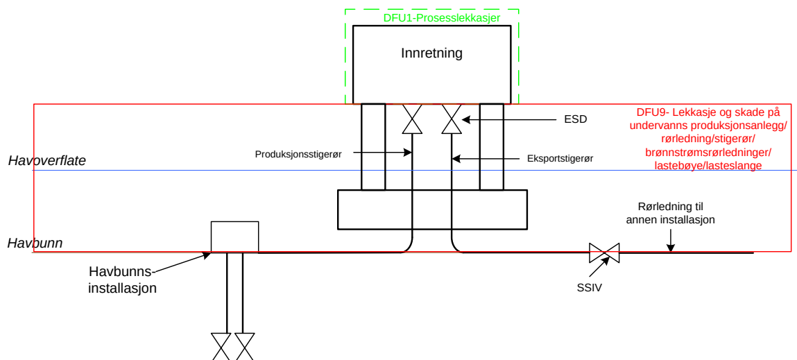
Figur 12 Skille mellom prosesslekkasjer (DFU1) og hendelser knyttet til undervanns produksjonsanlegg/rørledninger/stigerør/brønnstrømsrørledninger/lastebøyer/lasteslanger (DFU9-10)
